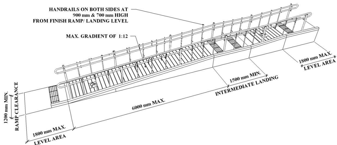
Fig. A.1.4 RAMP DIMENSIONS
